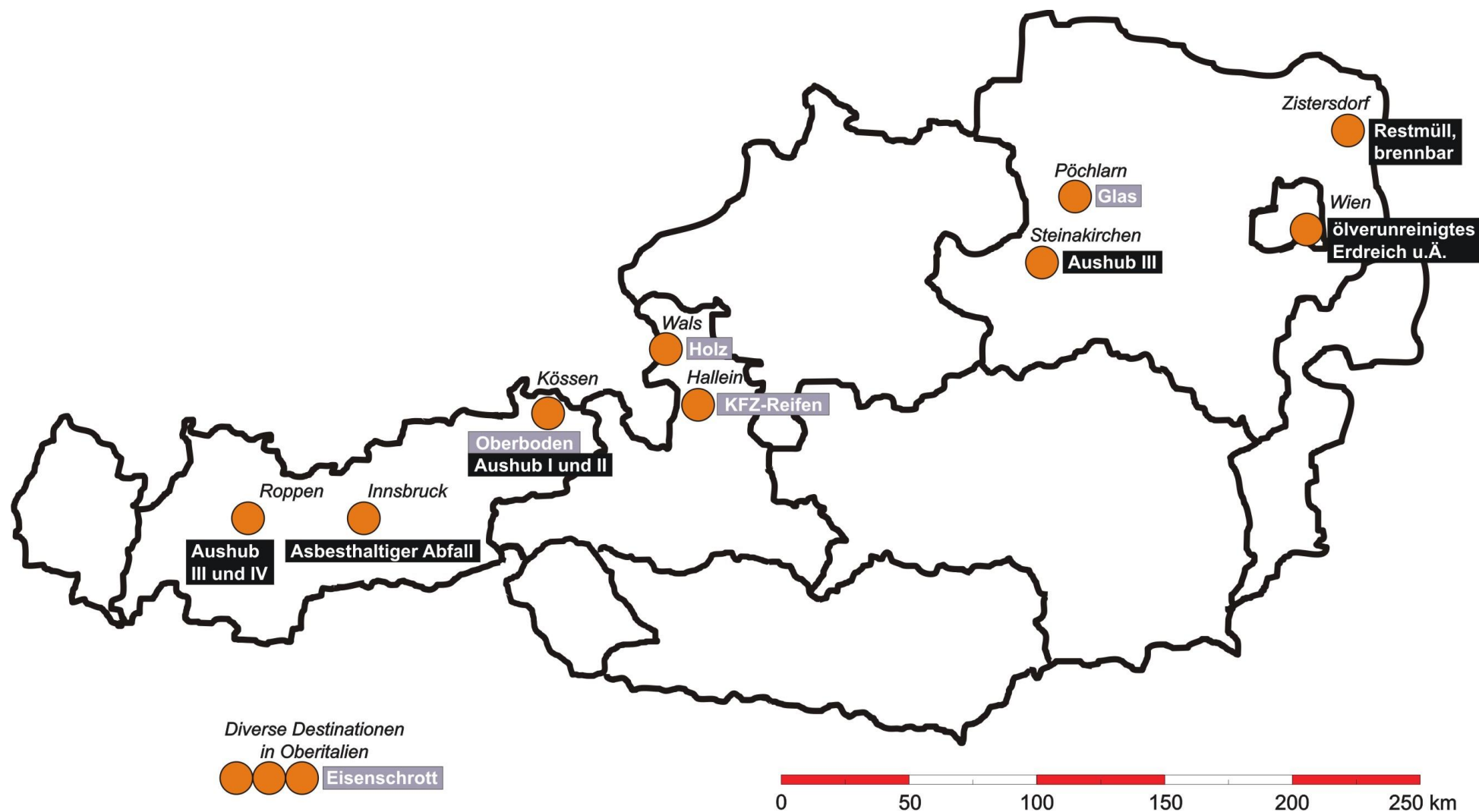
Abb. 58: Verwertungs- und Behandlungsdestinationen des „zerlegten“ Inhalts der Auwirtslacke: 70 % (dem Gewicht nach, bzw. 2/3 vom Volumen) verblieben in Kössen. Aushub I = Qualität Bodenaushub, Aushub II = Inertabfall, Aushub III = Baurestmassen, Aushub IV = Massenabfall.
