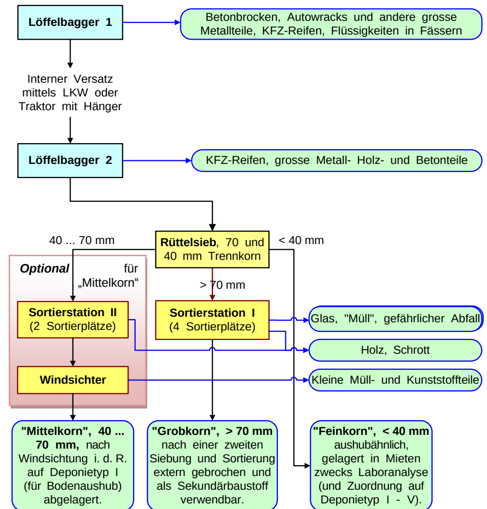
Abb. 28: Insgesamt angewendetes Aufbereitungsschema
