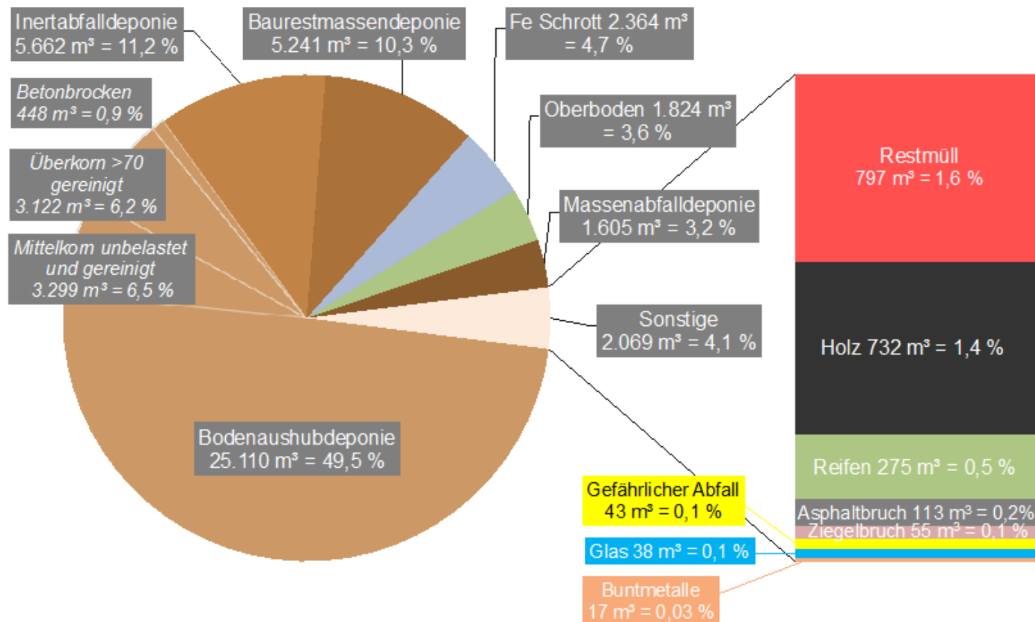
Abb. 47: Der Inhalt der Auwirlslacke – insgesamt 50.800 m 3 – in zerlegter Form: Volumensbilanz
