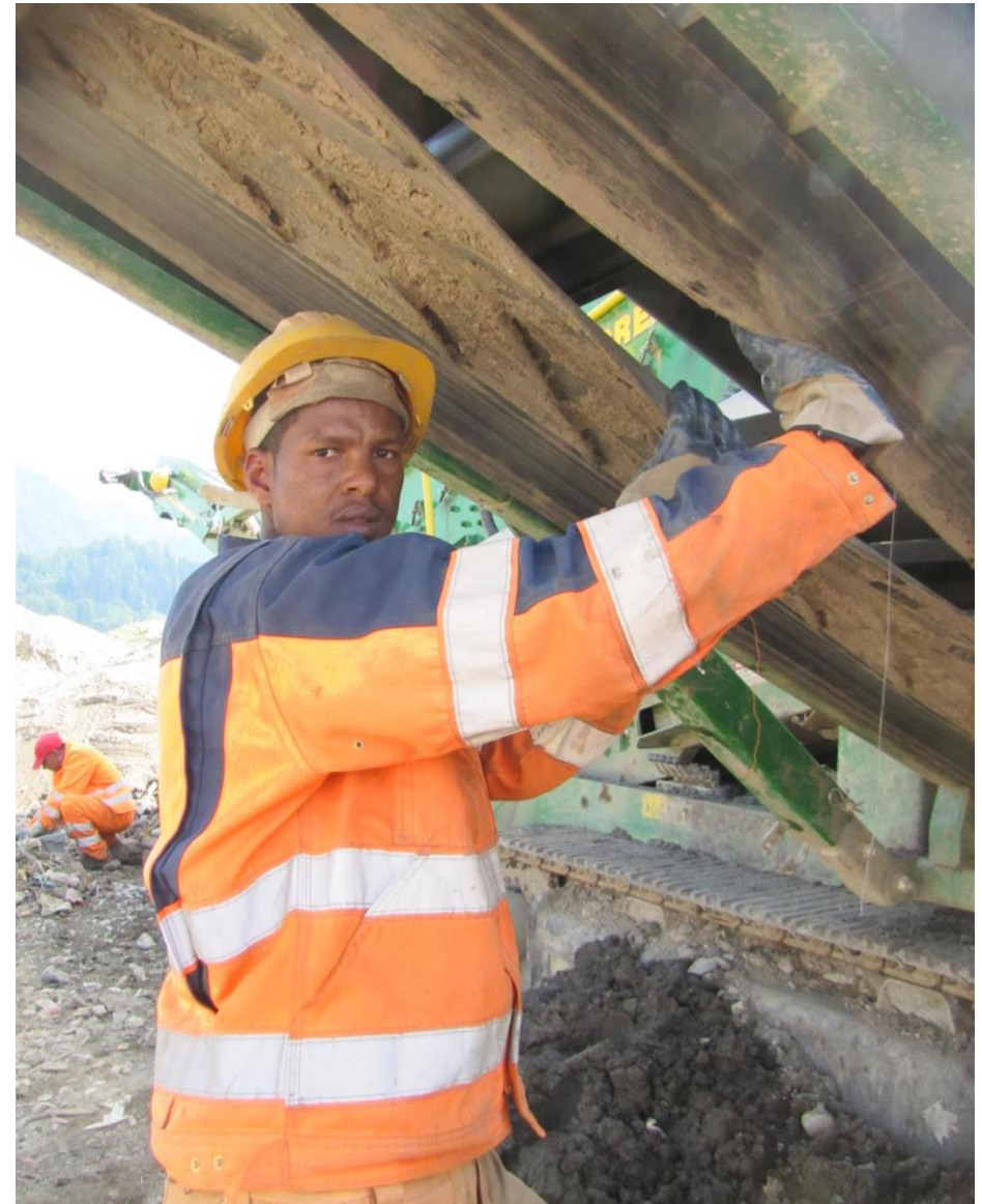
Abb. 55: Zerstörter Fördergurt (1. Juli 2015)
