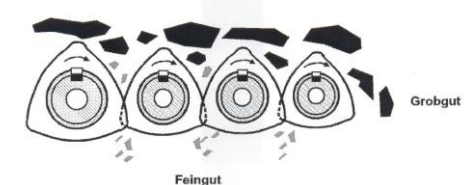
Abb. 17: Vier von fünf für die Siebung von Material mit den Eigenschaften des „Auwirtslacken“-Inhalts grundsätzlich zur Verfügung stehenden Gerätetypen ( Prinzipien nach Prof. Pretz, RWTH Aachen)
